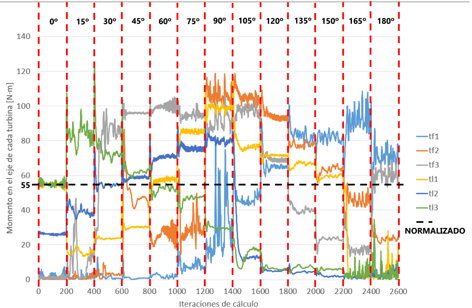
Gráfica de momentos en ejes de turbinas
