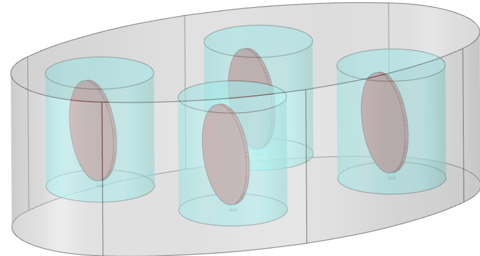
DISTRIBUCIÓN DE 4 TURBINAS AL TRESBOLILLO
