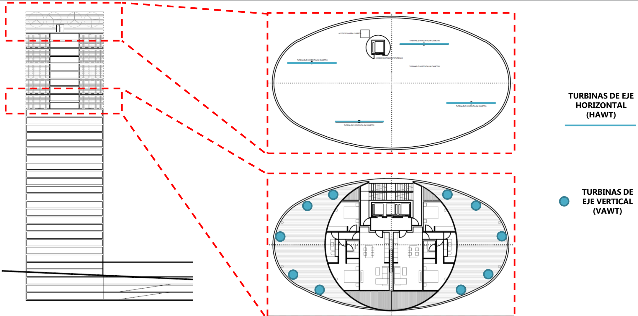
Geometría y esquema de distribución del edificio
