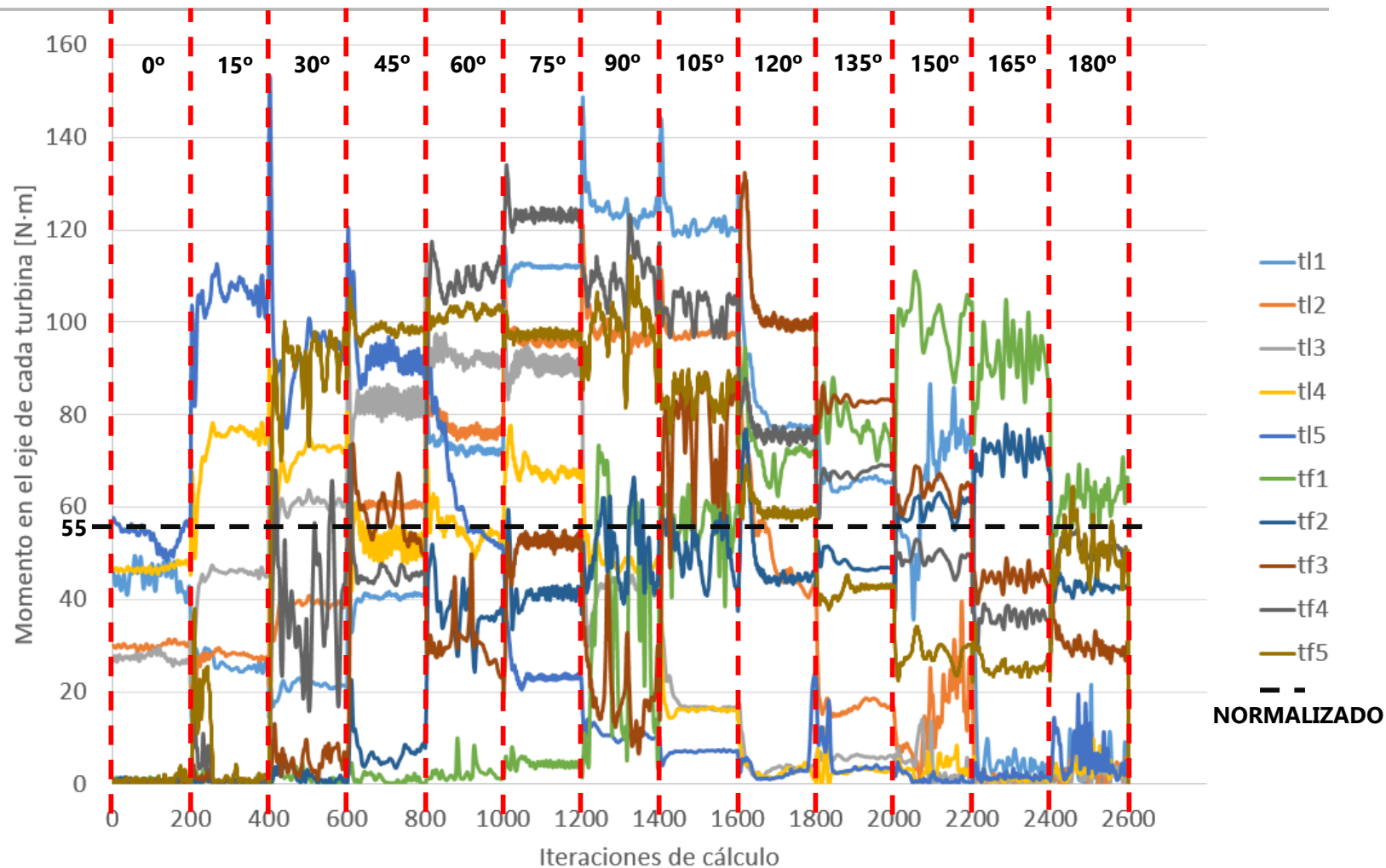
Gráfica de momentos en ejes de turbinas
