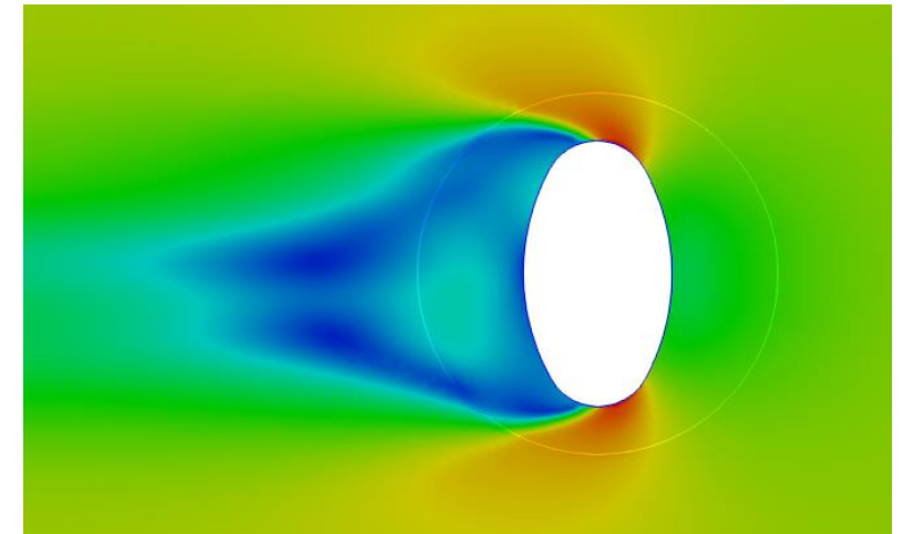
VIENTO INCIDENTE A 90°
